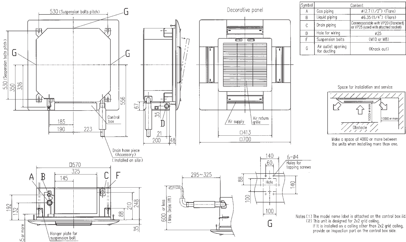
Модель FDTС40VF, 50VF, 60VF
