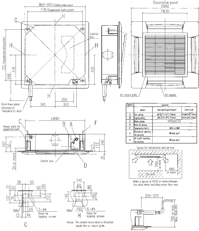
Модель FDTС40VF, 50VF, 60VF
