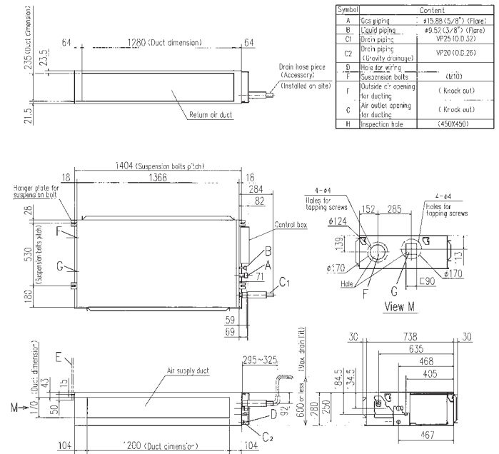
Модель FDU100VF1, 125VF, 140VF
