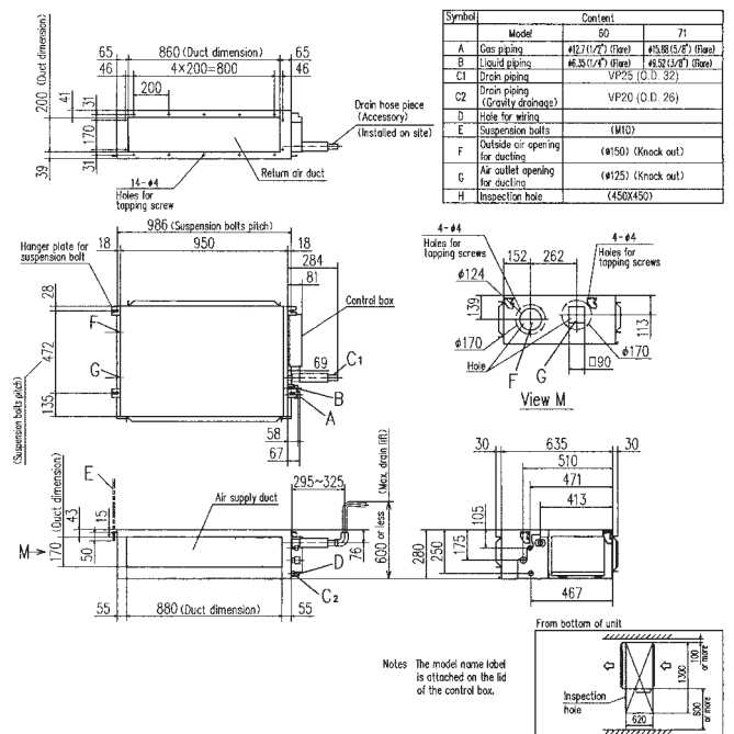
Модель FDUM60VF, 71VF
