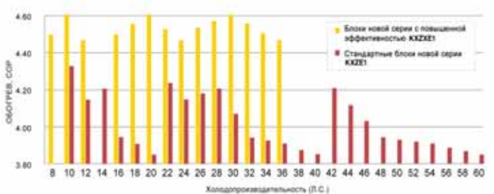
Сравнение коэффициента энергоэффективности стандартных блоков KXZ и блоков с повышенной энергоэффективностью
